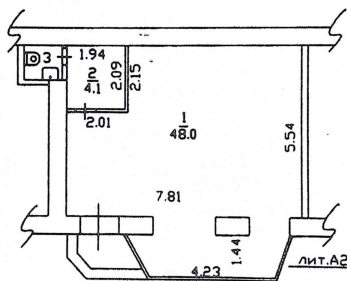
План строения лит.А-1 этаж нежилое помещение IV
