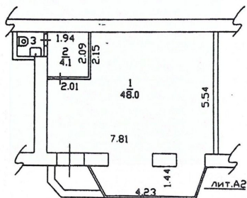
План строения лит.А-1 этаж нежилое помещение IV
